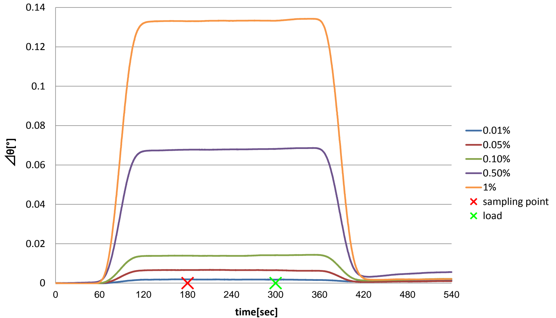
グルコース応答センサグラム
