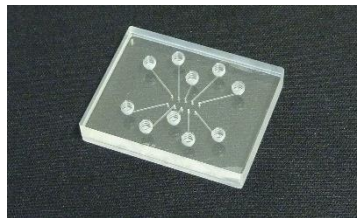
小型センサチップ用 フローセル押え板 (5ch型) 型式:MH-FCPR01-5C
