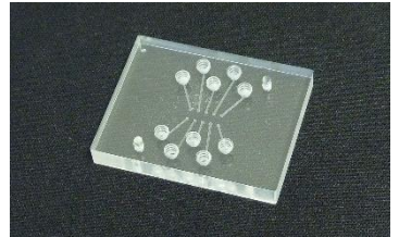
センサチップ用 フローセル押え板 (5ch型) 型式:MB-FCPR01-5C
