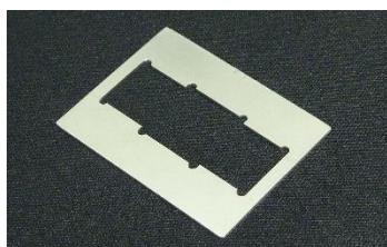
小型センサチップ用 PDMSフローセル位置合わせ板 型式:MH-FCAJ01
