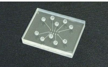
小型センサチップ用 フローセル押え板 (5ch型) 型式:MH-FCPR01-5C
